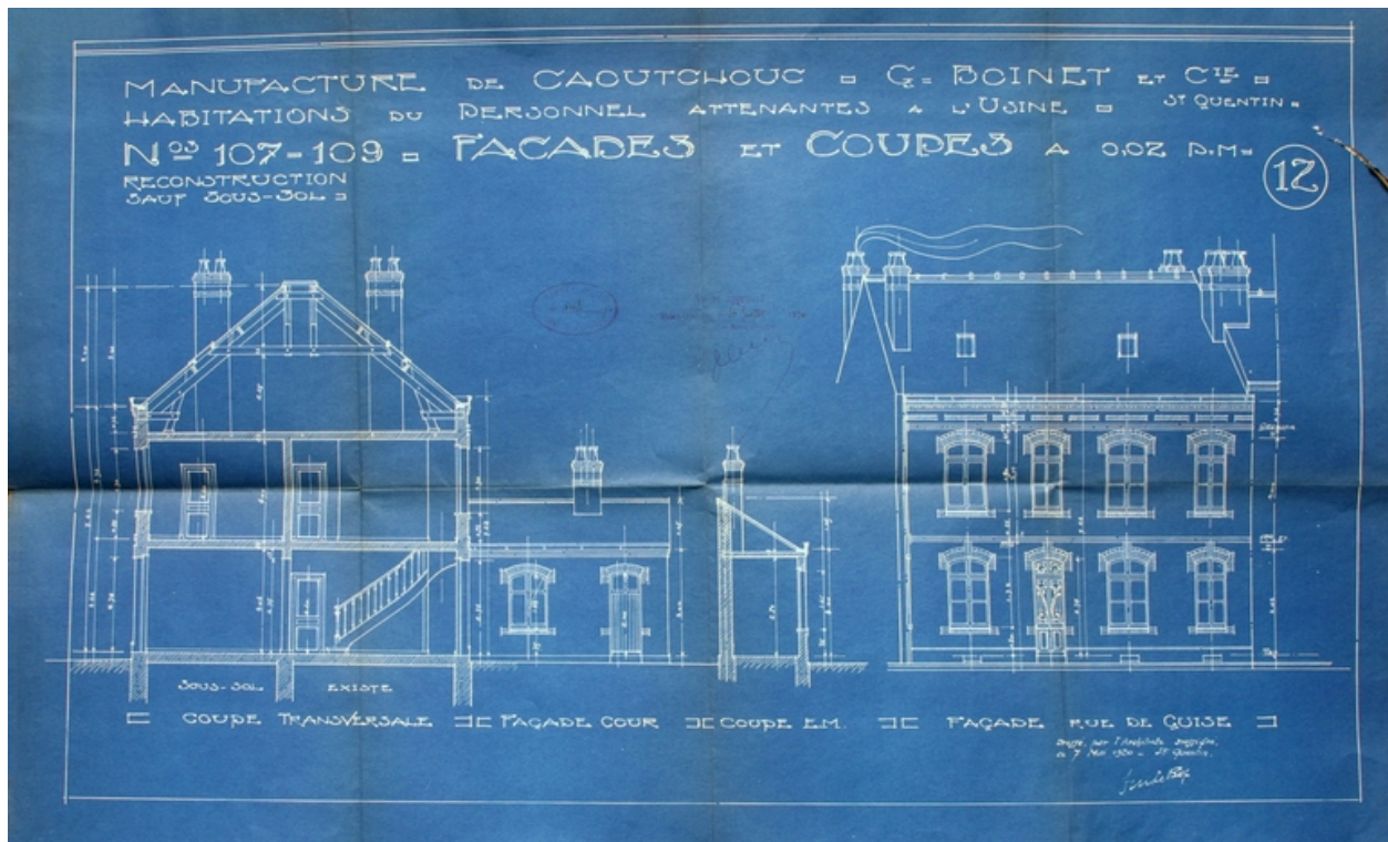
Coupe et façade antérieure d'une habitation rue de Guise, par Le Bot, 1920 (AC Saint-Quentin).
