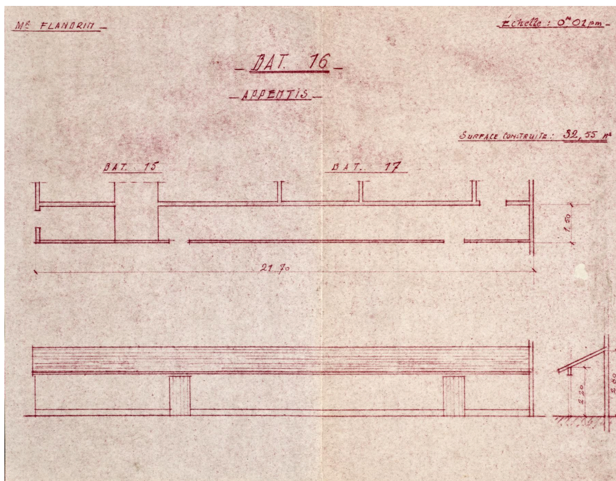
Plan, élévation, coupe d'un appentis, dressé par l'architecte Roger Pachot, [s.d.] (AD Somme, 1275 W 103).
