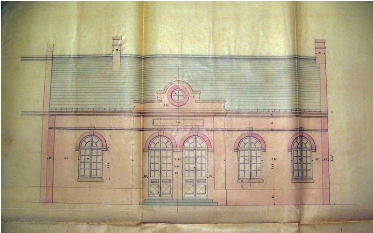
Façade par Caron, 1894 (AD Somme ; 99 O 710).
