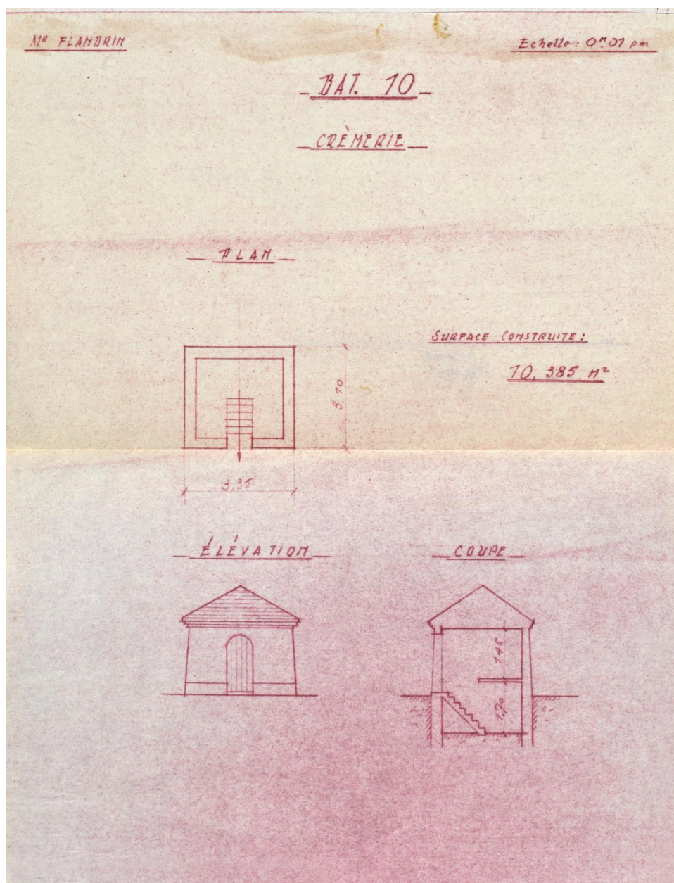
Plan, élévation, coupe de la crèmerie, dressé par l'architecte Roger Pachot, [s.d.] (AD Somme, 1275 W 103).
