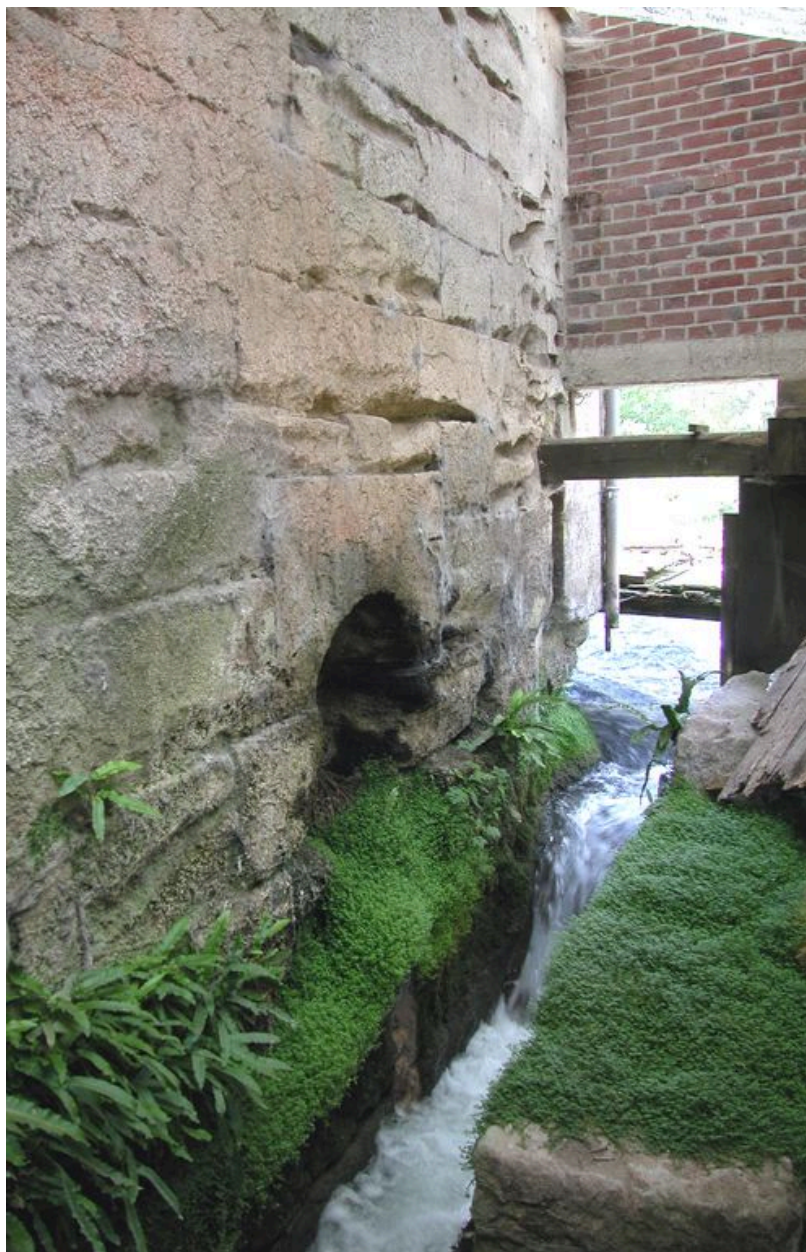
Vue intérieure de la cage du moulin, détail du coursier.
