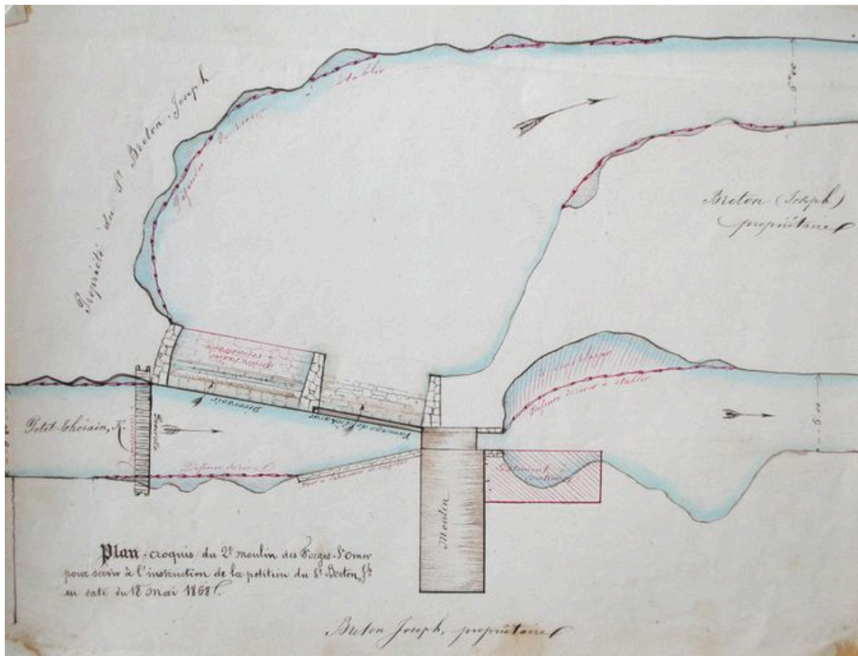
Plan du deuxième moulin des Forges appartenant à Joseph Breton, avec indication de la partie à construire, 18 mai 1868.
