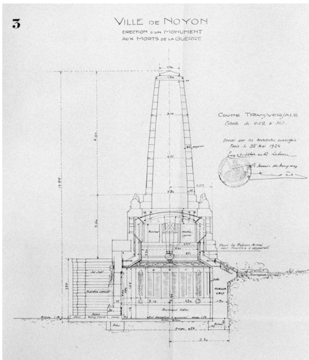
Coupe transversale, par E. Chifflet et R. Lefevre, 1924 (AD Oise ; série O).
