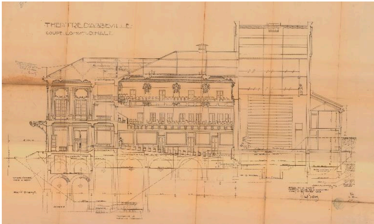
Coupe longitudinale, tirage, par Paul Bessine, 25 janvier 1912 (AD Somme ; 99 O 35).
