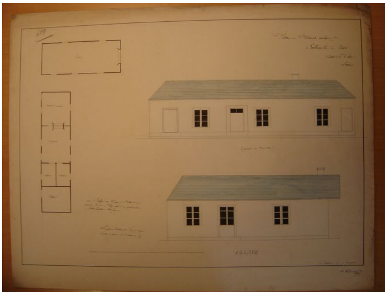
Plan et élévation de la première école de Salenelle vers 1870.
