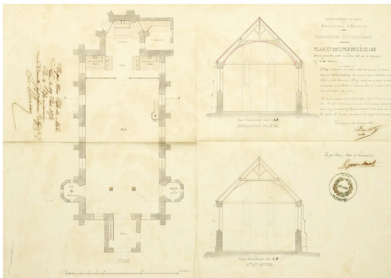
Plans et coupes de l'église, 1851 (AD Nord).
