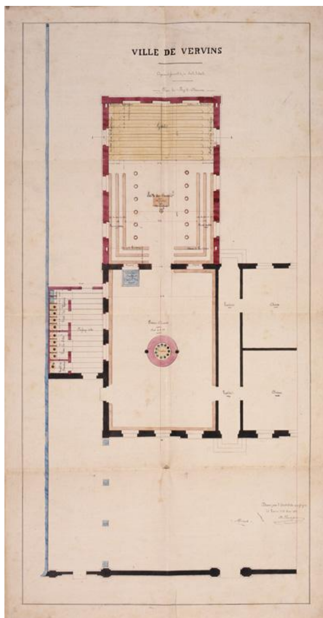
Plan d'un projet d'extension sur l'arrière, non suivi d'exécution, 1868.
