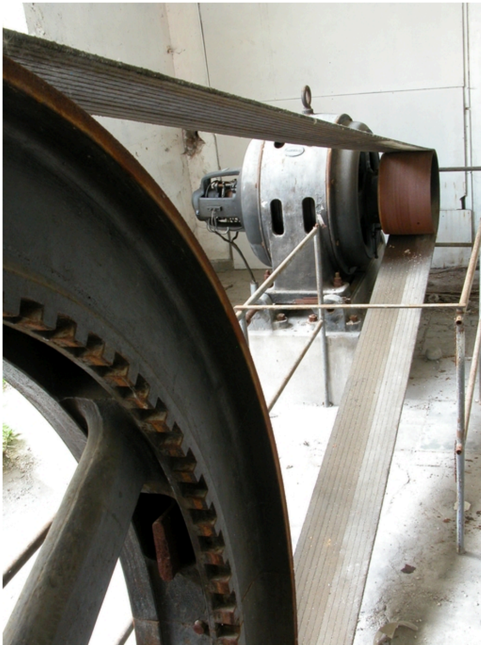
Le volant et sa courroie de transmission, reliée au groupe générateur.
