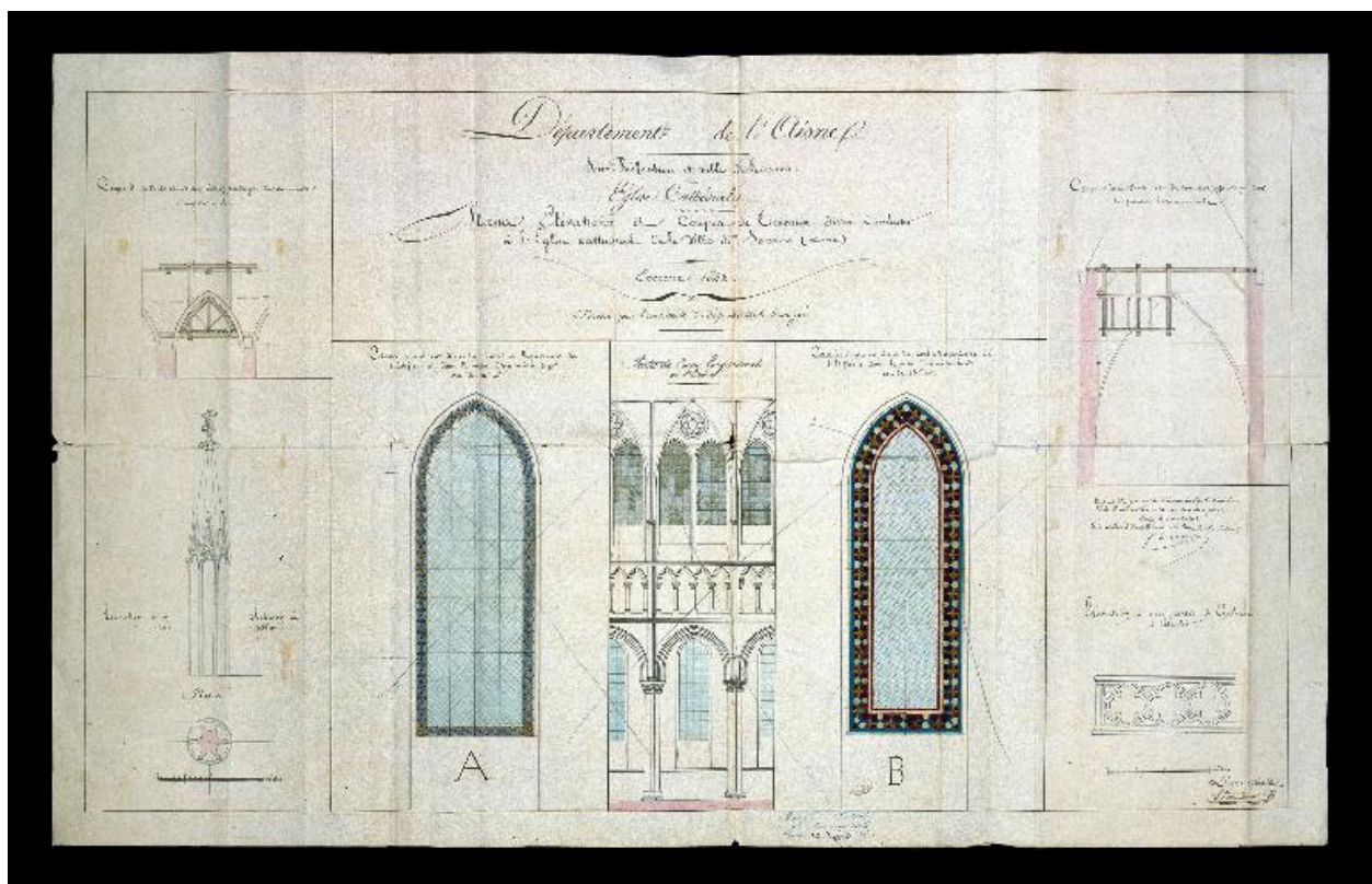
Plans, élévations et coupes de travaux à exécuter à la cathédrale de Soissons au cours de l'exercice 1842, dessinés par l'architecte départemental Henri van Cléemputte (AN : F 19, carton 7887).
