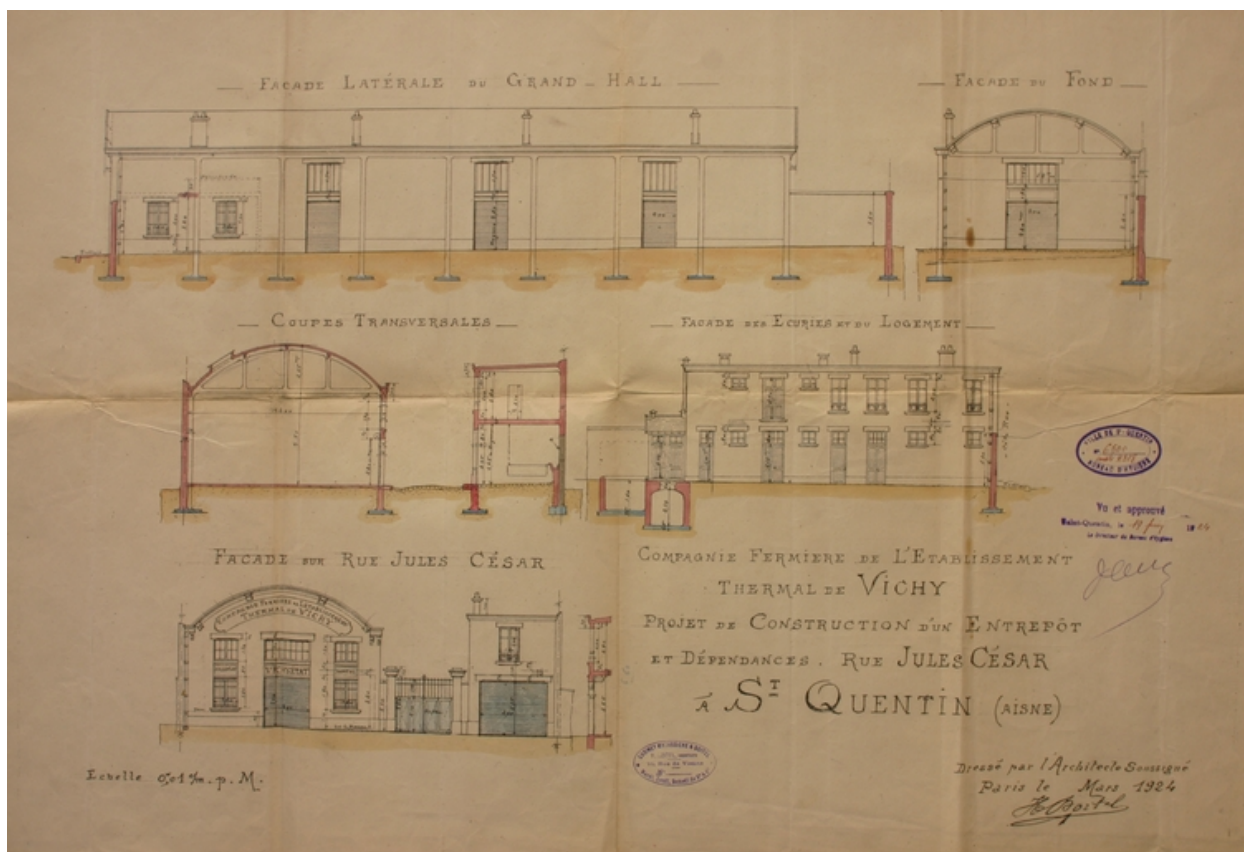
Façades et coupes, par Boitel, 1924 (AC Saint-Quentin).
