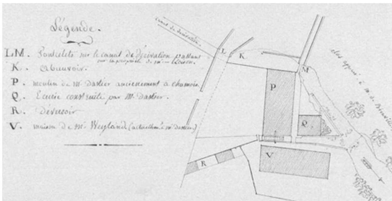
Usine IV : le moulin à chamois est transformé en moulin à blé, 1809 (AD Oise ; 7SP293).
