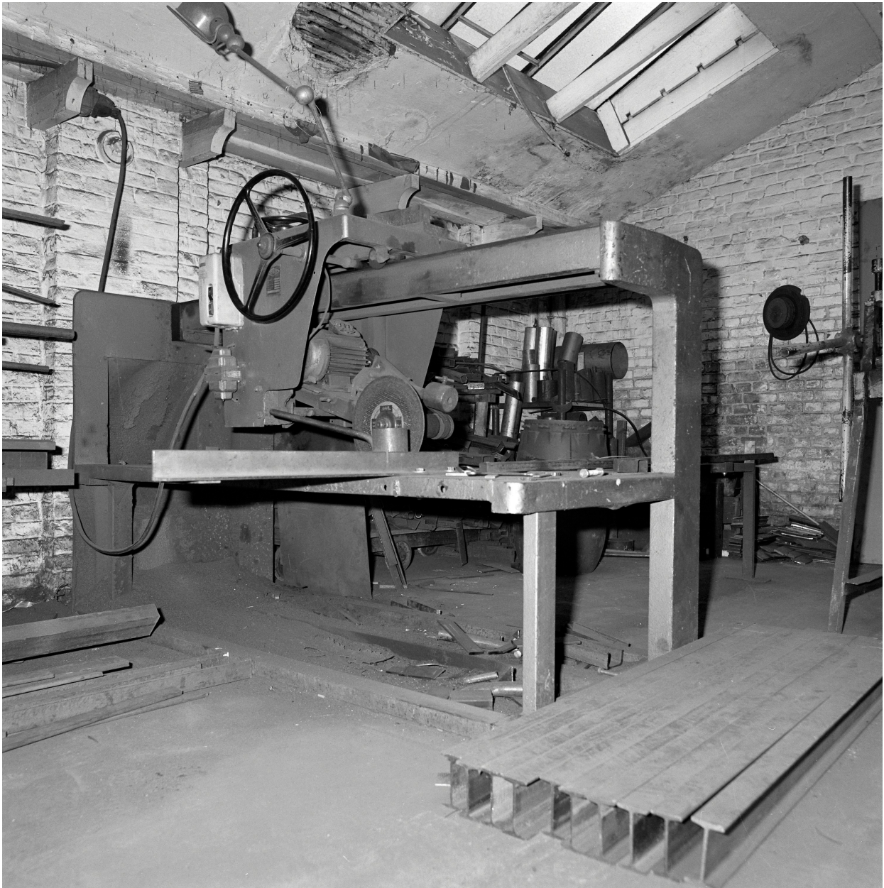
Atelier de fabrication, tronçonneuse (sans marque).
