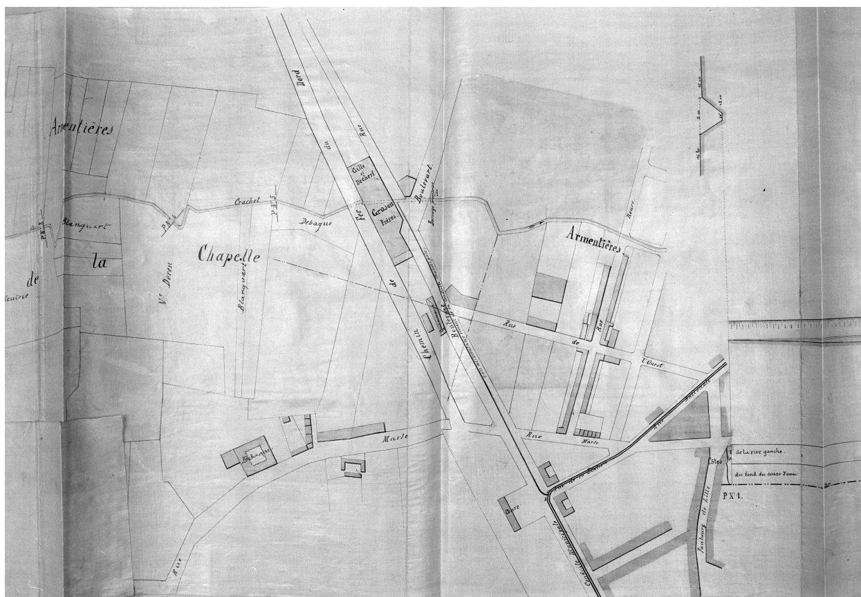
Filature Gruson. Plan de situation et du réseau d'eau, 1873 (AD Nord ; S 3788).
