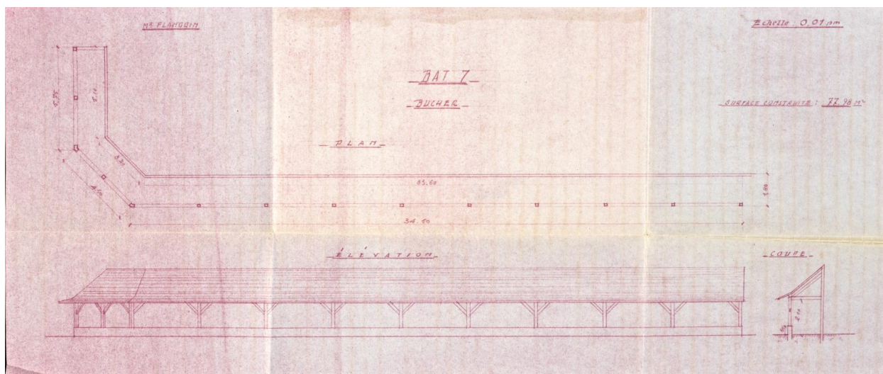
Plan, élévation, coupe du bucher, dressé par l'architecte Roger Pachot, [s.d.] (AD Somme, 1275 W 103).
