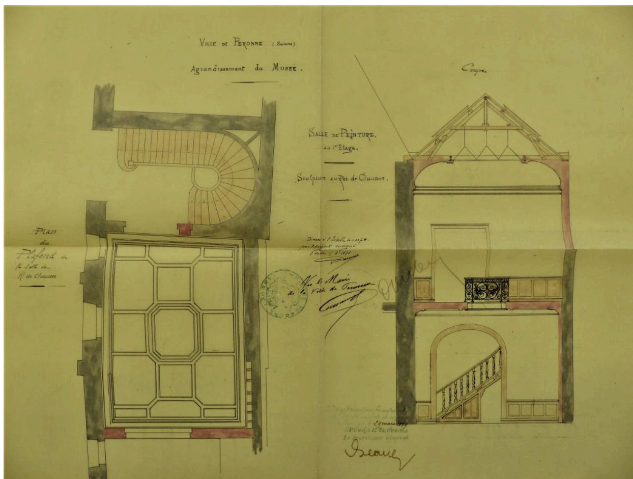
Ville de Péronne. Agrandissement du musée. Plan et coupe. Omer Darcourt architecte, 1898 (AD Somme ; 99O 2998).
