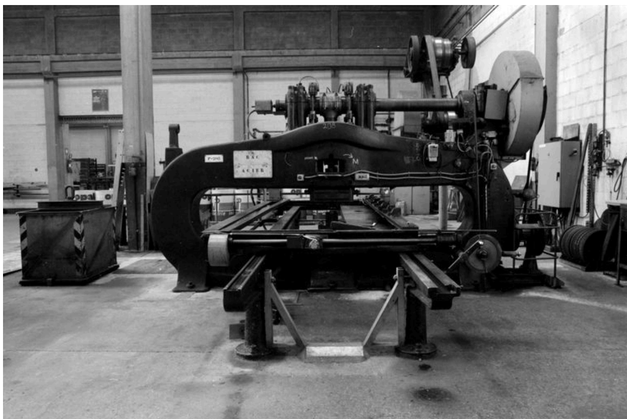
CLAIROIX. Usine d'emboutissage Gantois. Machine de production.
