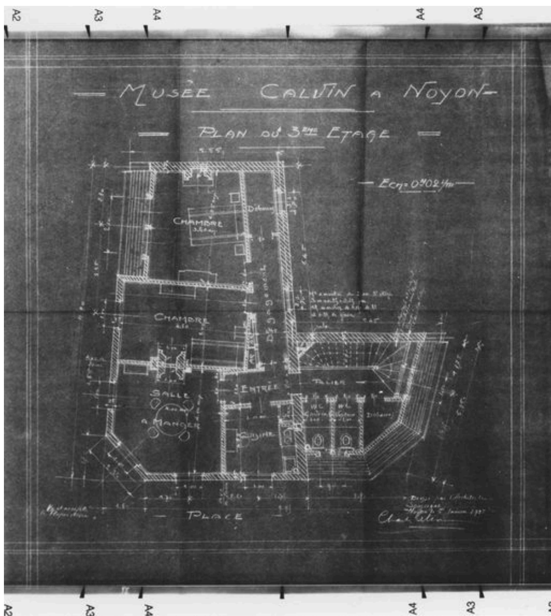
Plan du 3e étage. Projet de restauration, par Letrosne, 1927 (AC Noyon).
