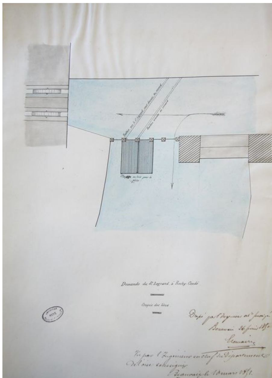
Plan partiel du système hydraulique du moulin appartenant à M. Adam et exploité par Legrand, scieur d'os, par Lemaire (ingénieur des Ponts-et-Chaussées), 1851.
