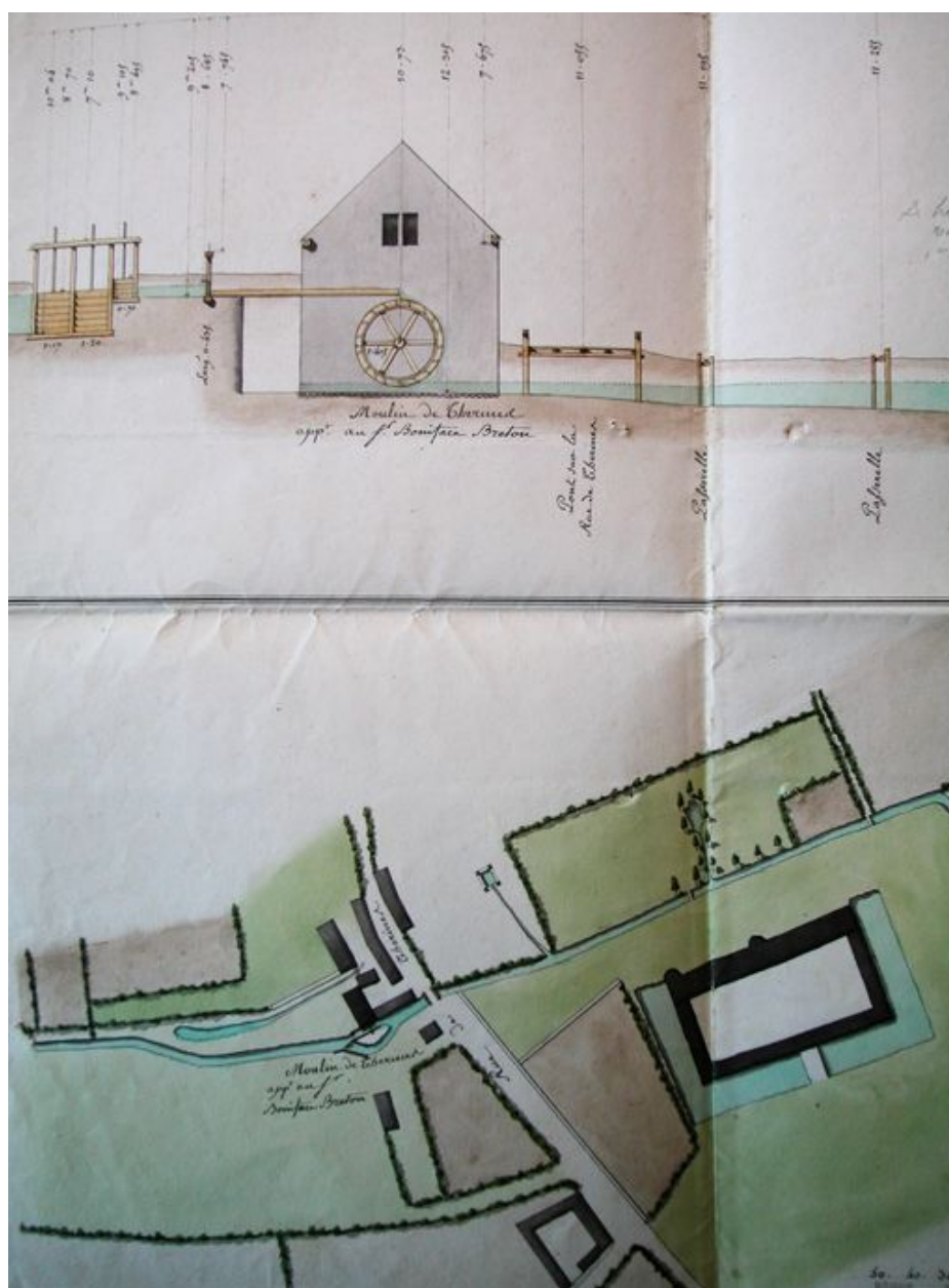
Plan et profil du moulin du sieur Boniface Breton, tel qu'il existait en 1813.
