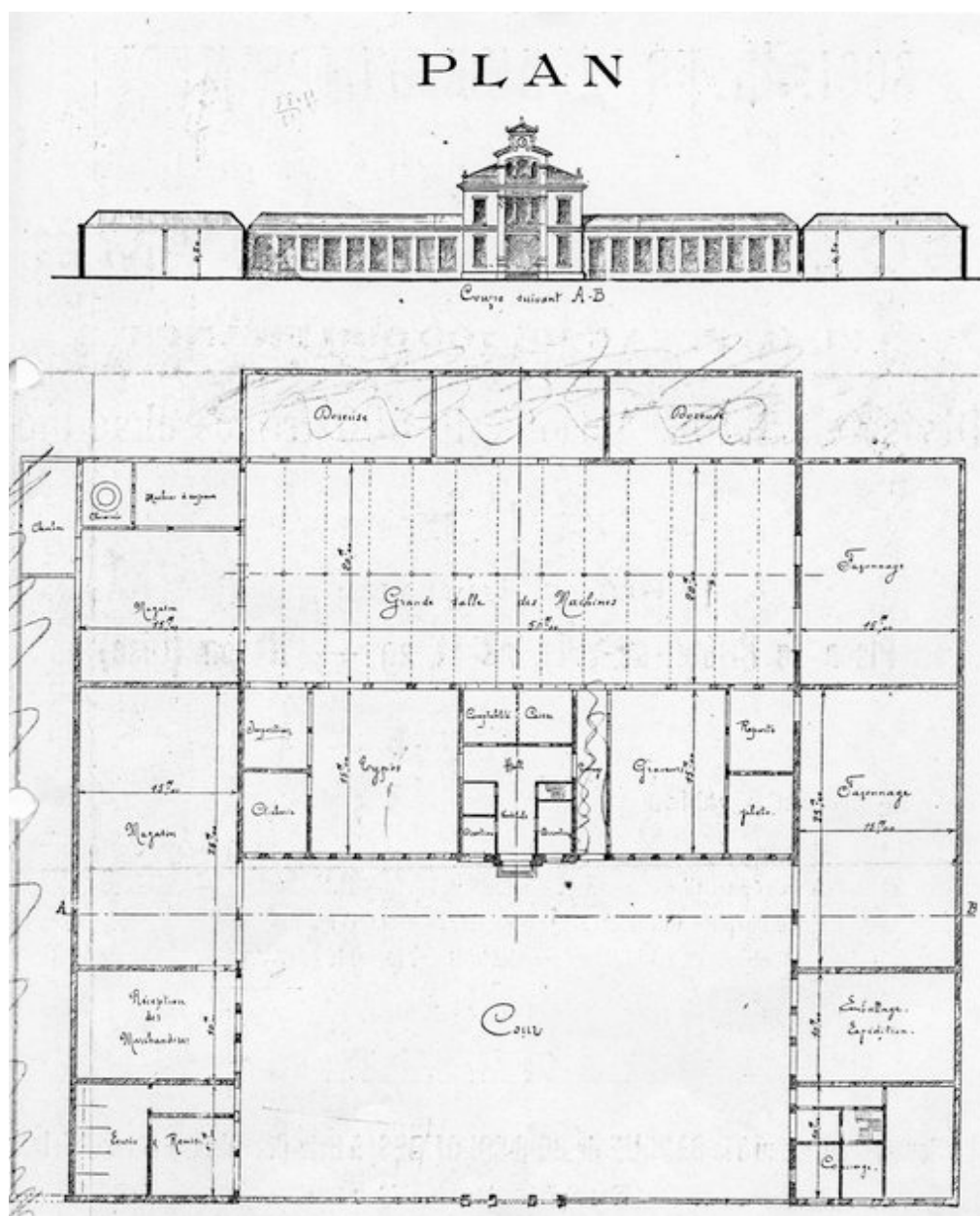
Plan et élévation d'une imprimerie (AD Oise ; fonds Silvert, 471-1895).
