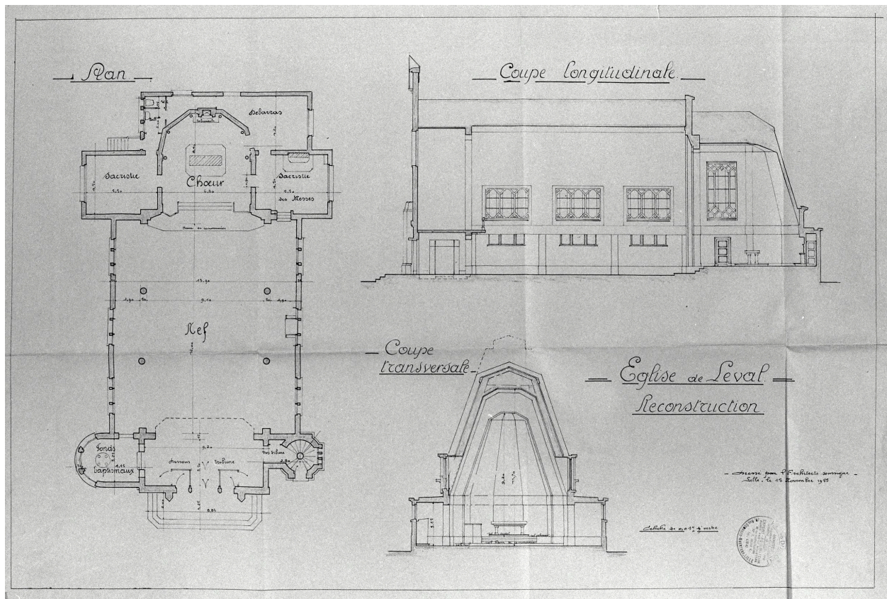
Plan, coupes longitudinale et transversale de la nouvelle église par Fernand Dumont (architecte communal), 15 novembre 1955 (AC Leval ; dossier église).
