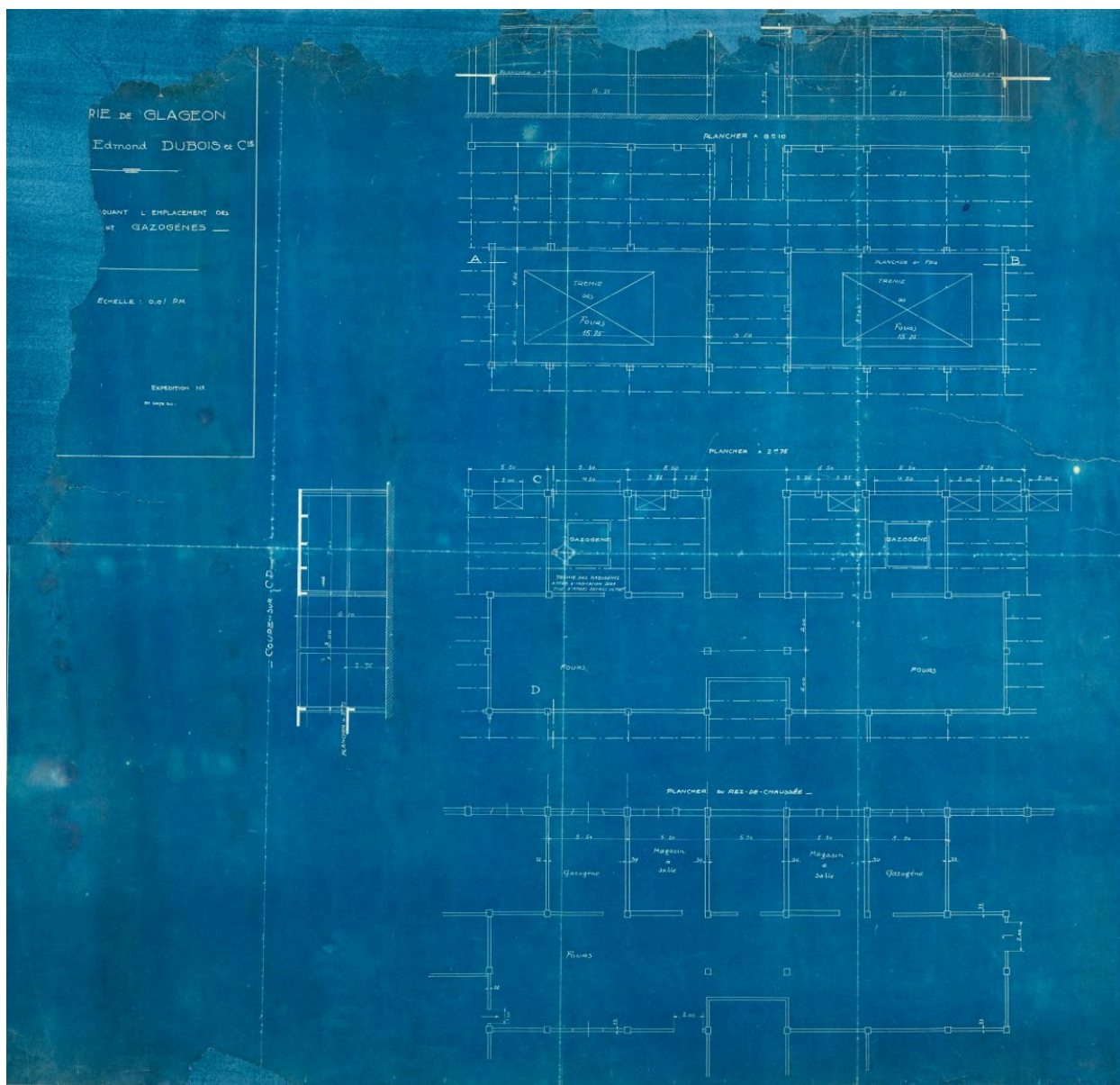
Verrerie de Glageon de MM Edmond Dubois et Cie. Plan des planchers et emplacements des gazongènes, non daté (circa 1920).
