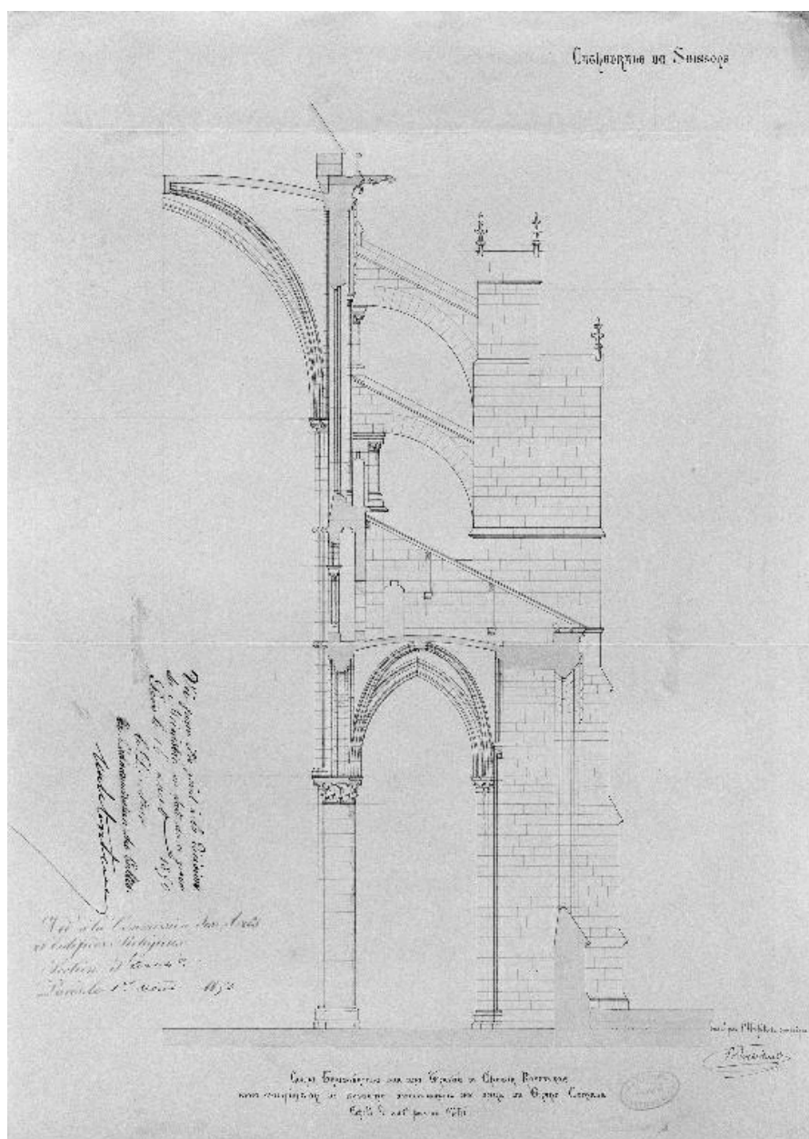
Coupe transversale sur une travée du chœur restaurée, avec modification du système d'écoulement des eaux du grand comble, dessinée par l'architecte Émile Boeswillwald en 1850 (AN : F 19 7887).
