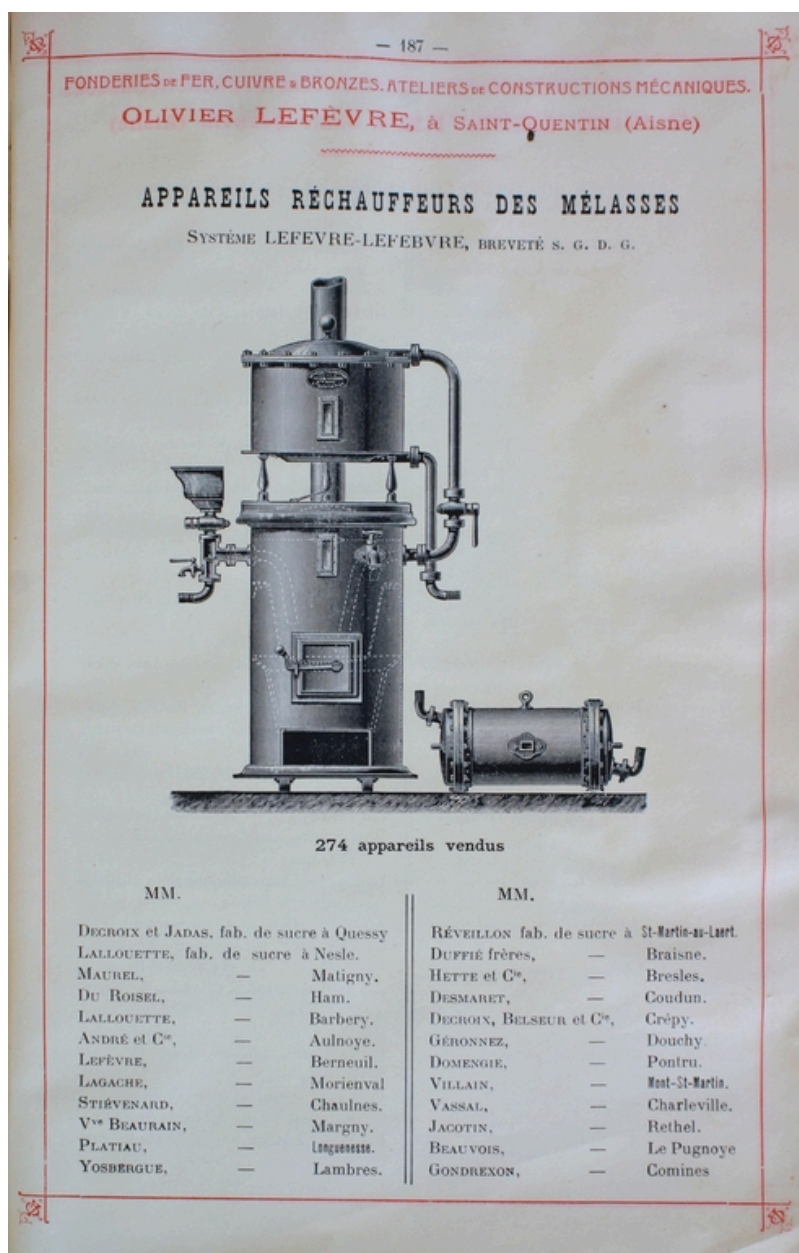
Appareils réchauffeurs des mélasses, 1902 (AC Saint-Quentin).
