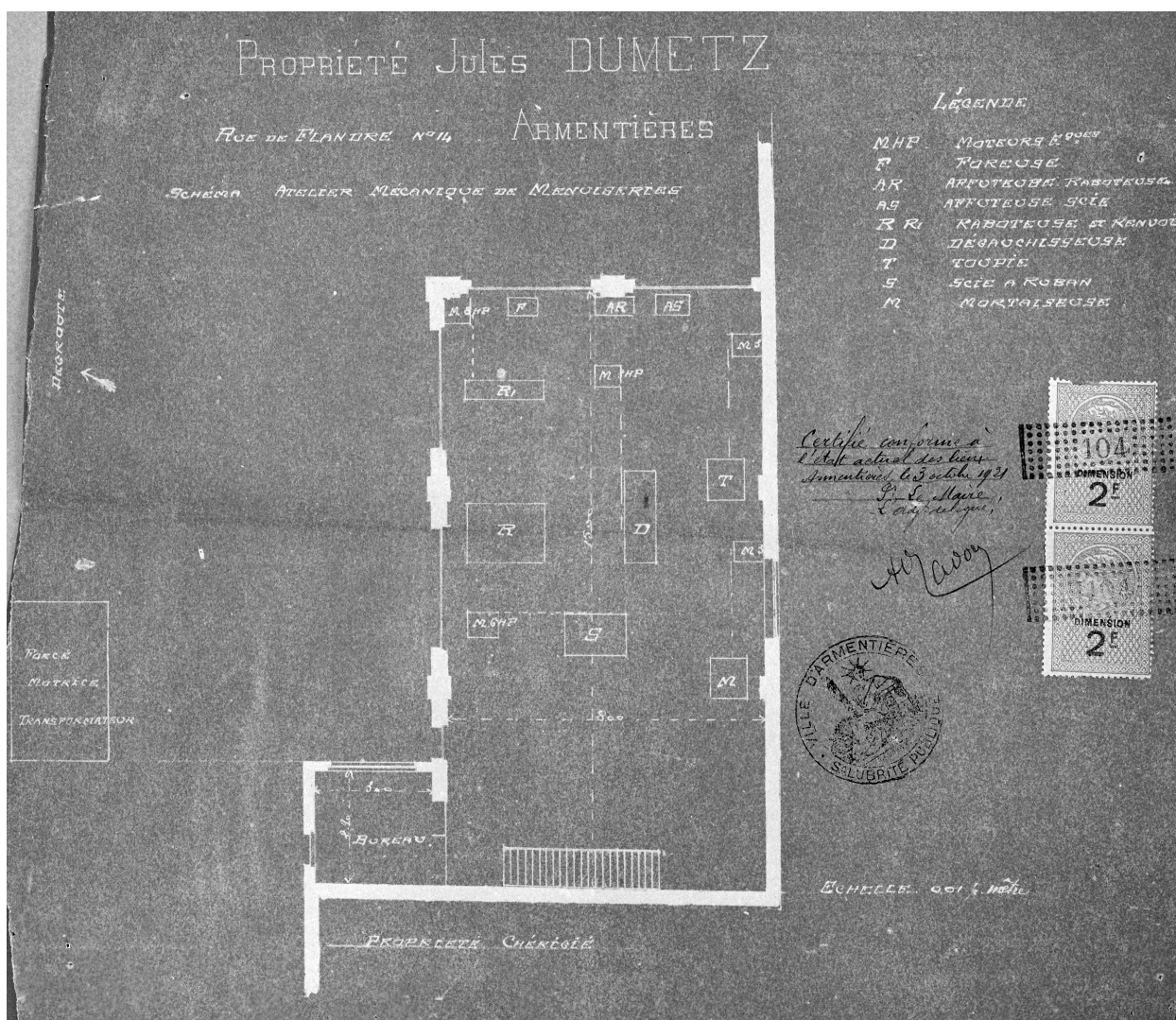
Installation de la scierie Jules Dumetz. Plan masse, 1921 (AD Nord ; M 41710347).
