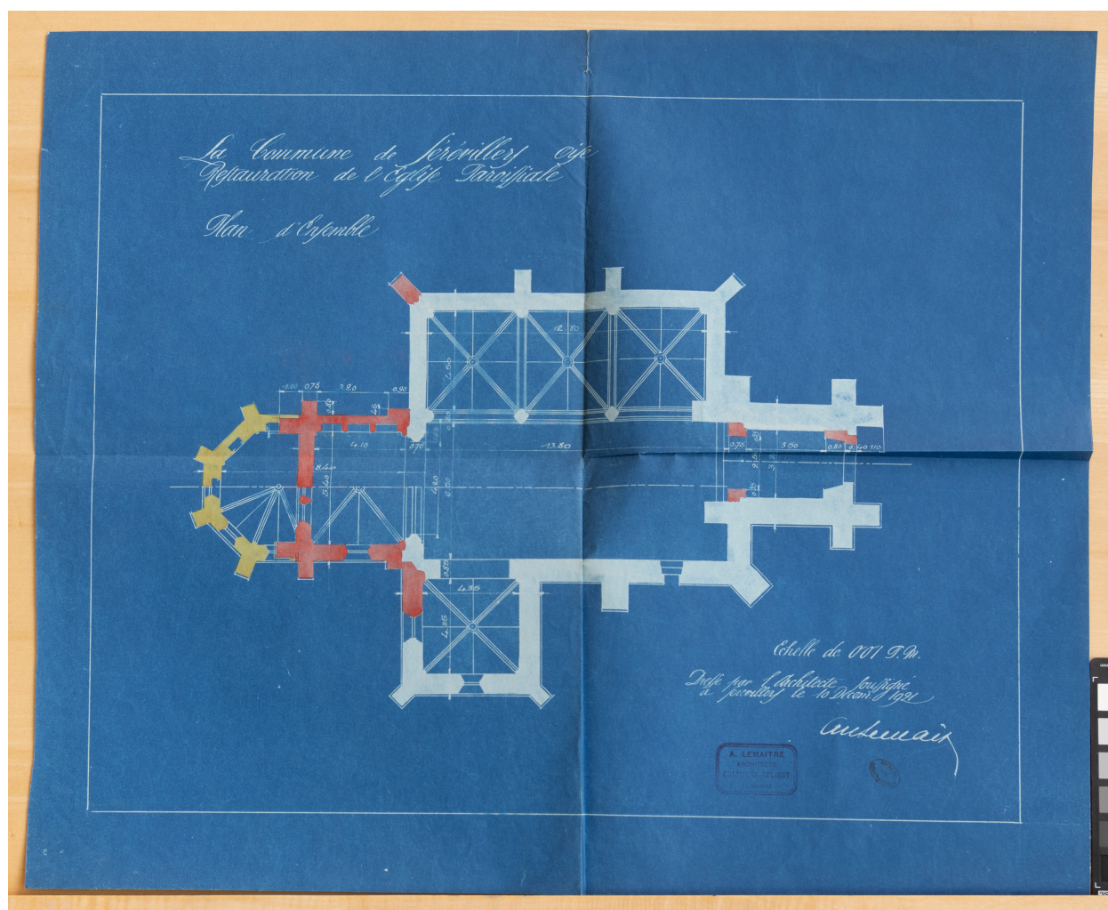
Église de Sérévillers (Oise). Plan au sol des parties détruites, par A. Lemaître, 1921 (AD Oise).
