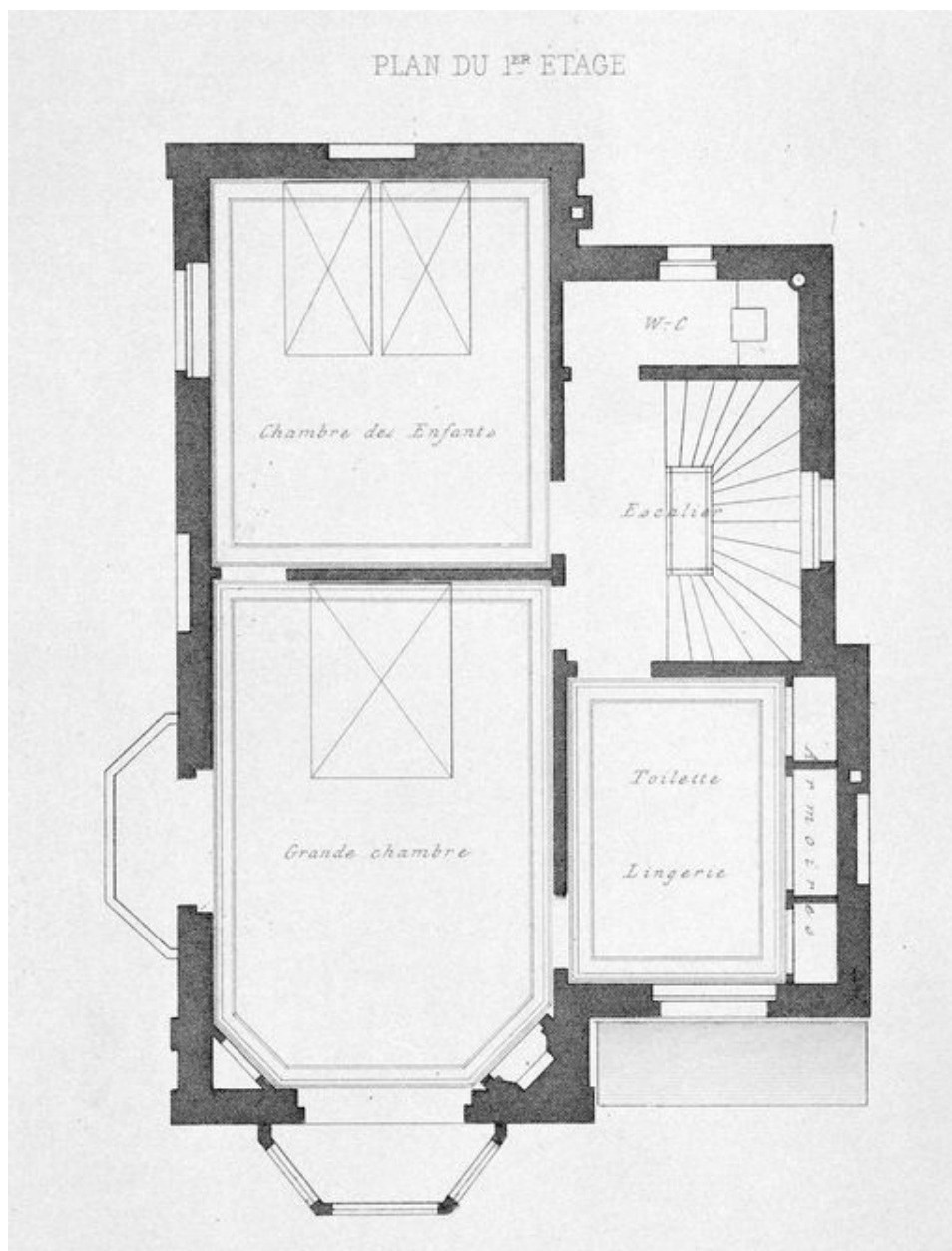
Villa Simplette, plan du premier étage (AD Somme ; 1 J 3596/9).
