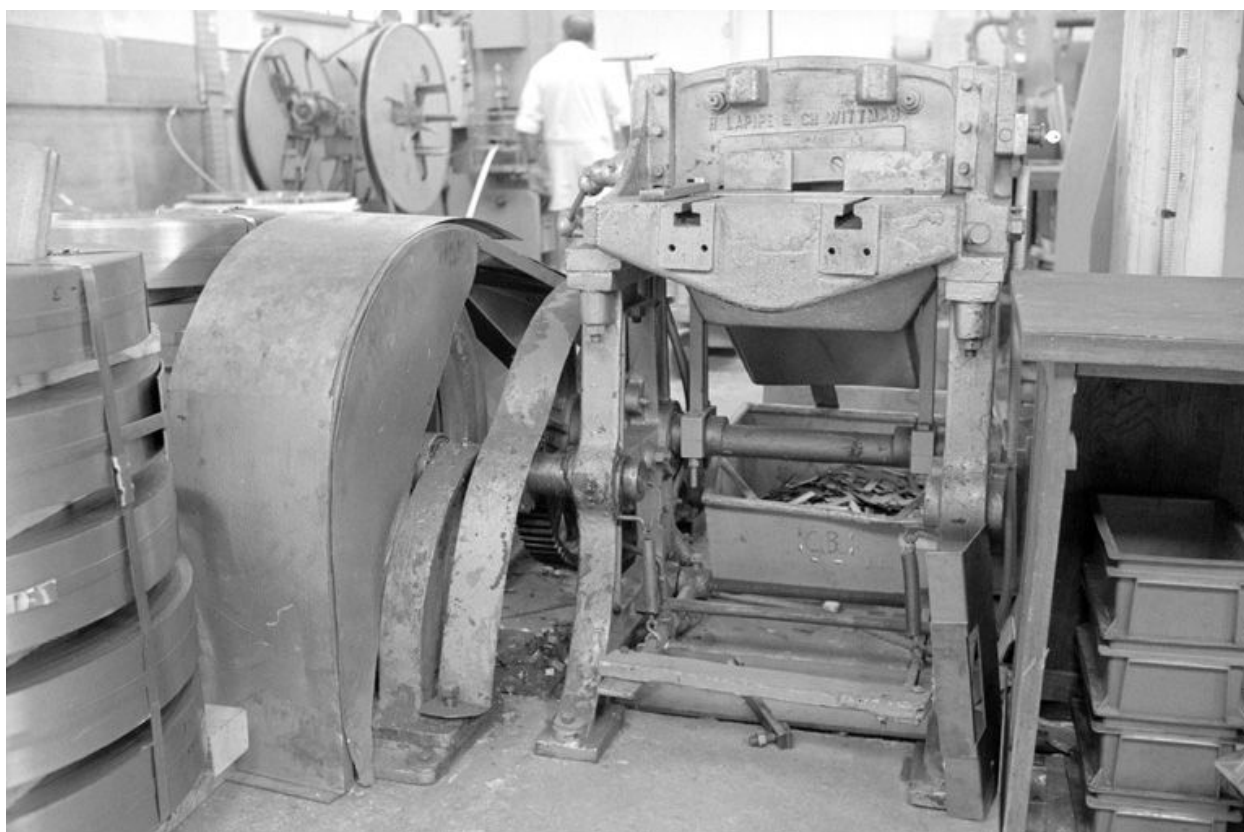
Atelier de fabrication, vue intérieure : cisaille H. Lappe et Ch. Wittmann 1924, en 1990.
