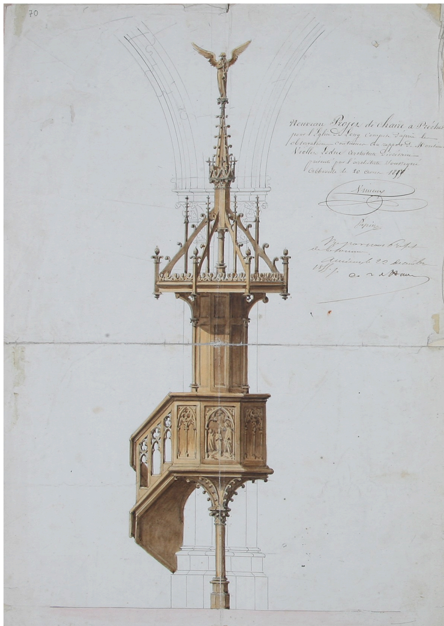
Nouveau projet de la chaire à prêcher suite au rapport de Viollet-le-Duc, dessin des frères Duthoit, 1855 (Archives du musée de Picardie, Duthoit, alb 18 fo 70).
