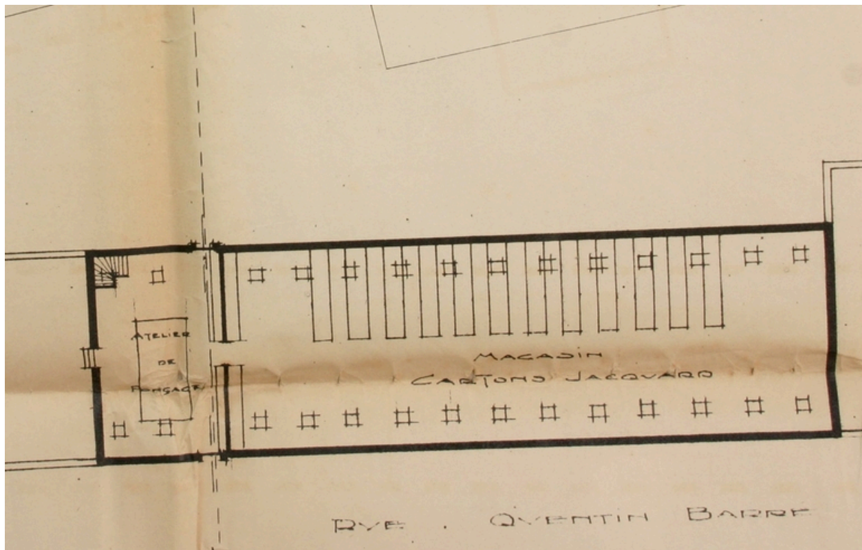
Plan du deuxième étage de l'usine Trocmé à la veille de la Première Guerre mondiale, dressé après 1919 par Chauquet, Navile et Christol. Détail (AD Aisne).
