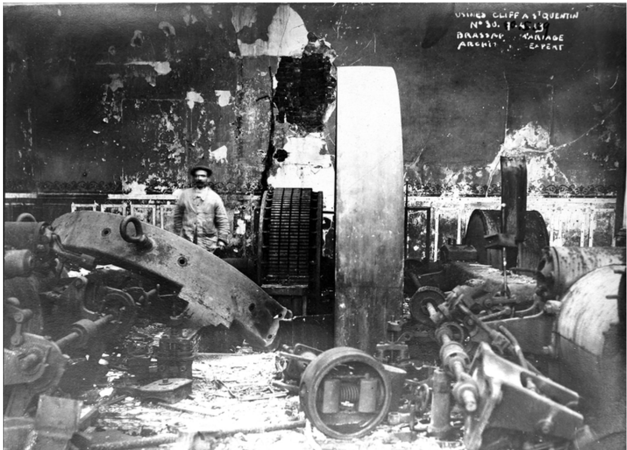
La machine à vapeur principale, par Brassart-Mariage, mai 1919 (AD Aisne).
