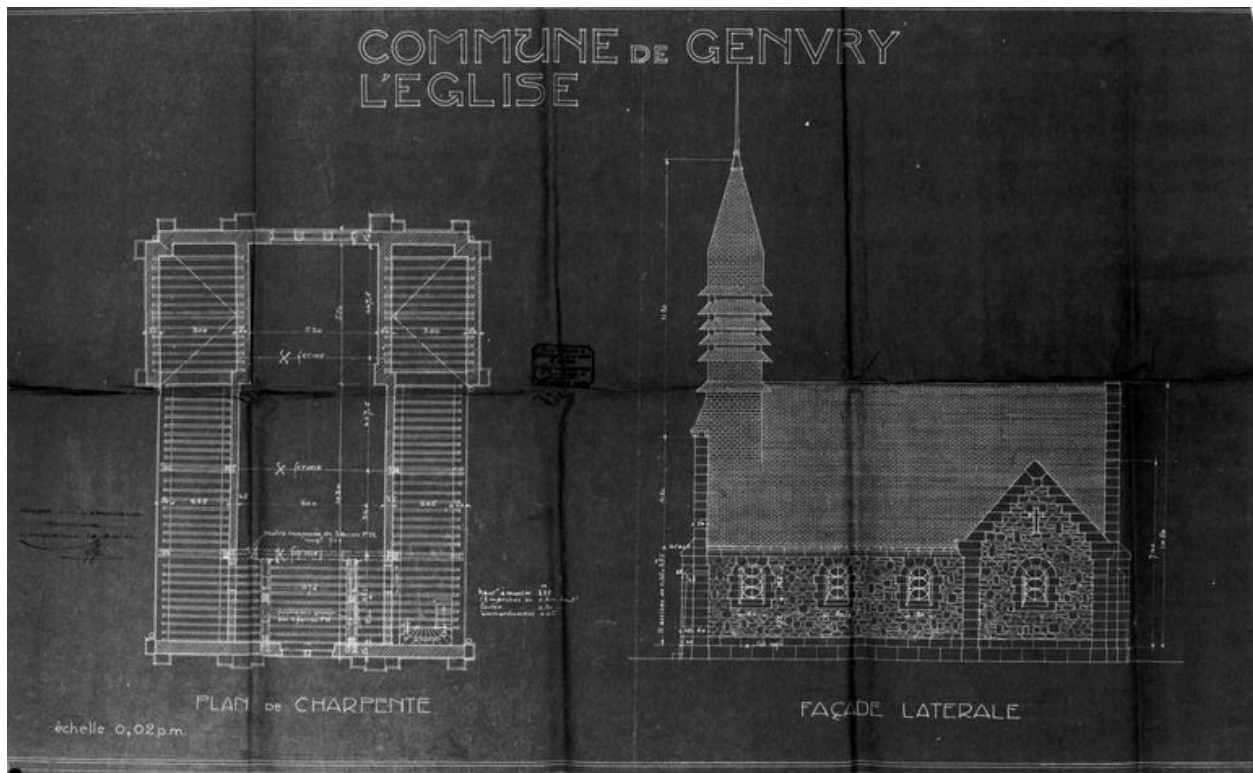
Plan de la charpente, élévation latérale, par M. Mages, 1923 (AD Oise ; série O).
