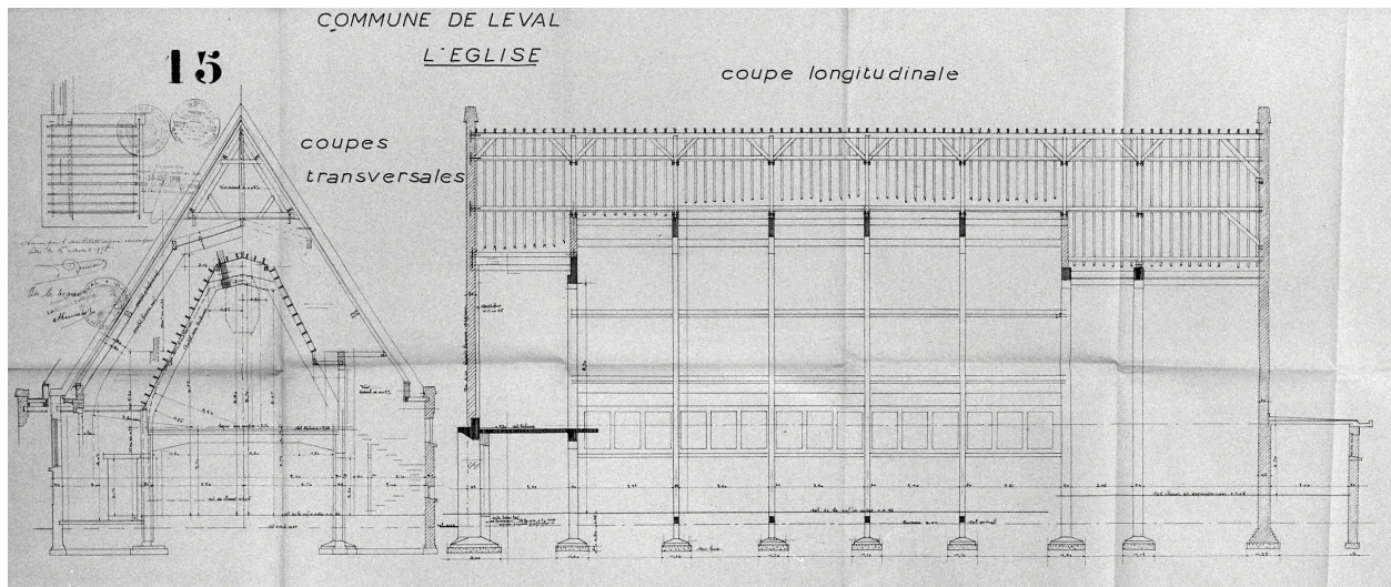
Coupes transversale et longitudinale de la nouvelle église. Plan de Fernand Dumont (architecte communal), 6 août 1959 (AC Leval ; dossier église).
