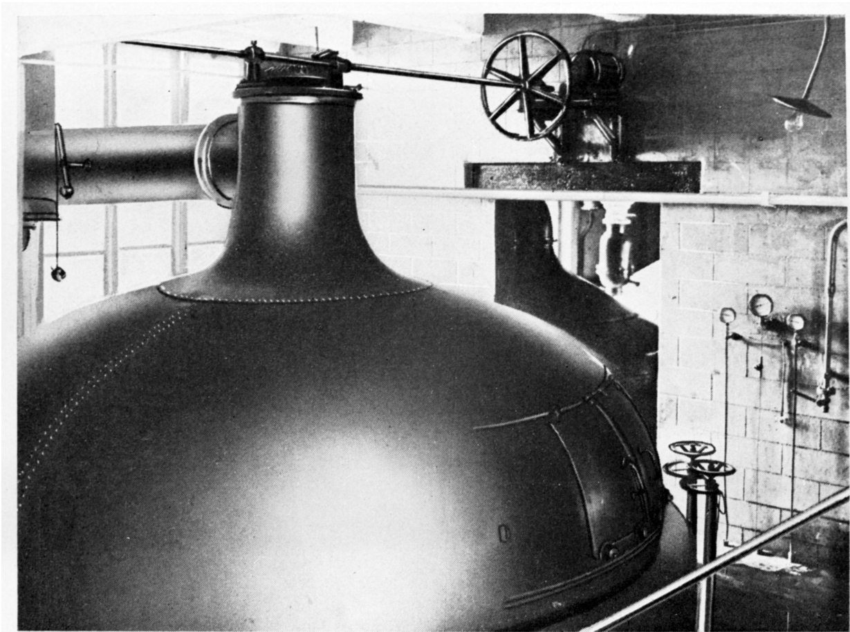
UNE DES CHAUDIÈRES DE BRASSAGE (MEURA)
