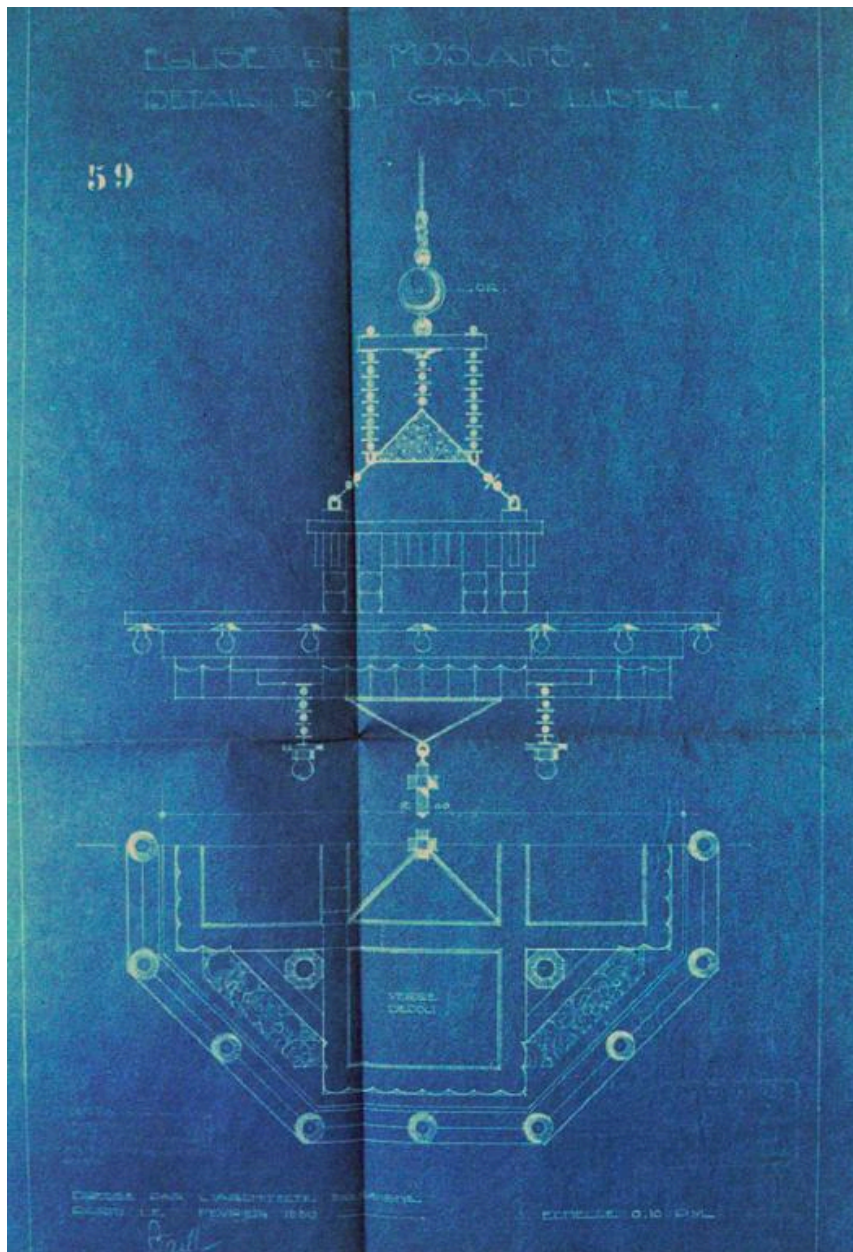
Détail du grand lustre, Louis Faillé (architecte), février 1930 (AD Somme ; 99 o 2676).
