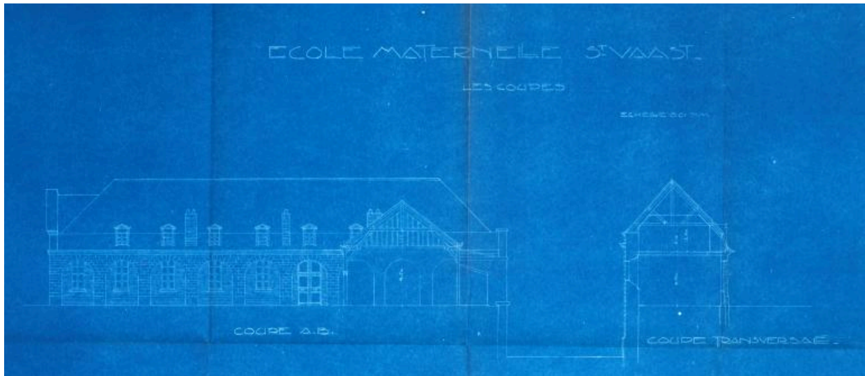
Arras. École maternelle Saint-Vaast. Les coupes. État vers 1920 (AD Pas-de-Calais ; 10R 4).
