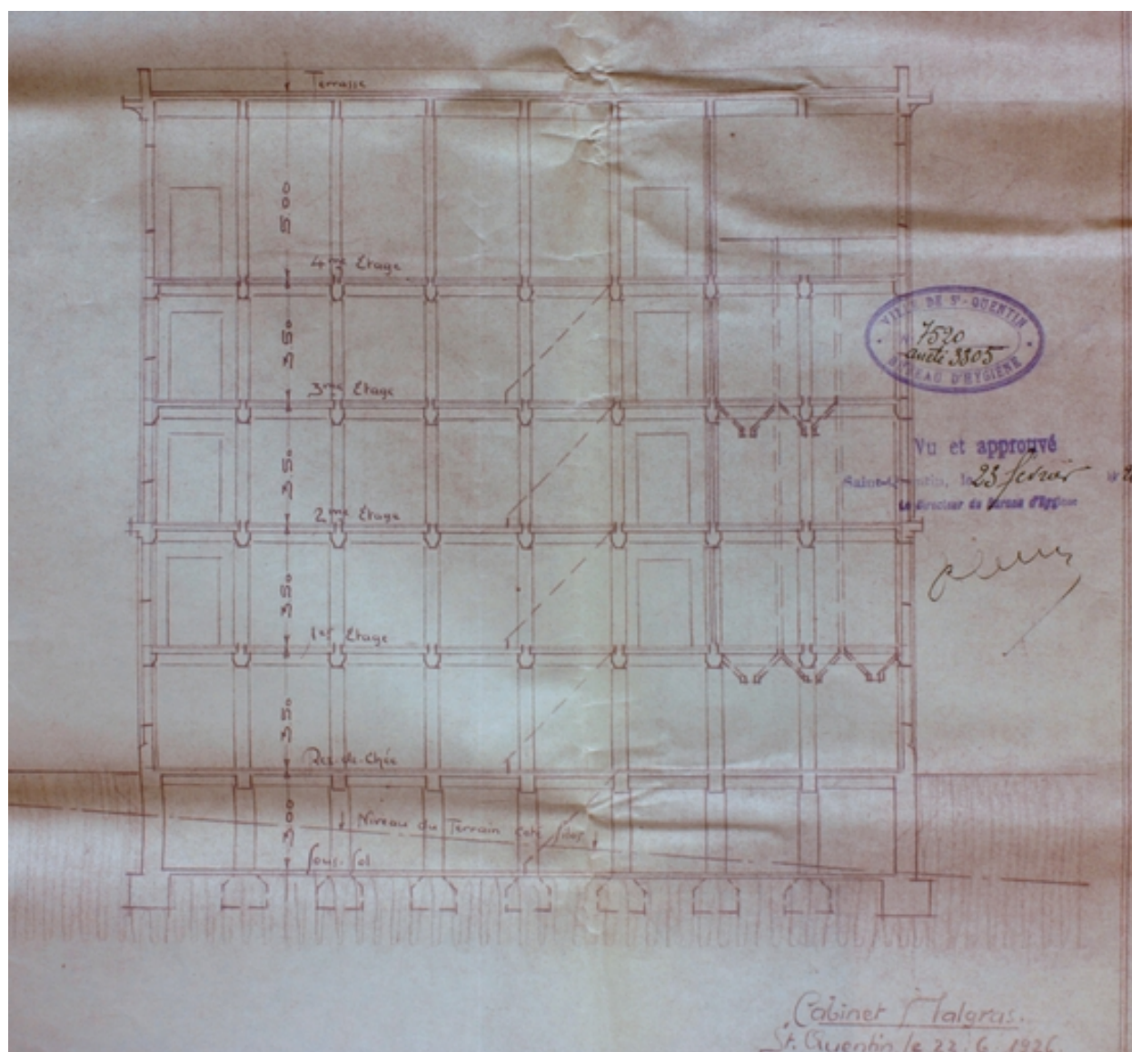
Coupe transversale de la minoterie, par Magras-Delmas, 1926 (AC Saint-Quentin).
