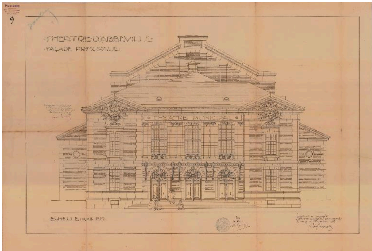
Élévation de la façade principale, tirage, par Paul Bessine, 25 janvier 1912 (AD Somme ; 99 O 35).
