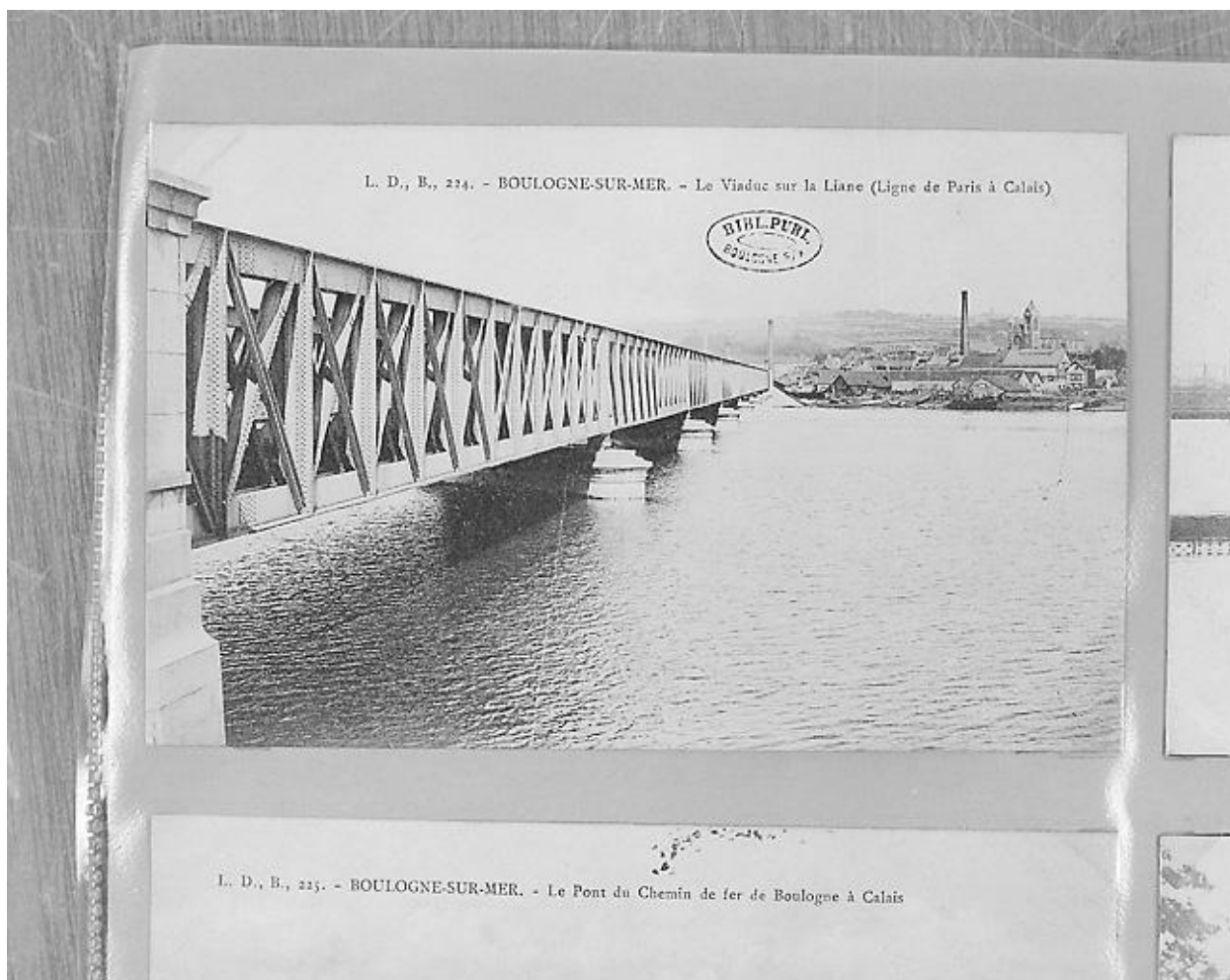
Pont métallique dit viaduc, vue de profil en amont, carte postale. B.M. Boulogne-sur-Mer, collection cartes postales.
