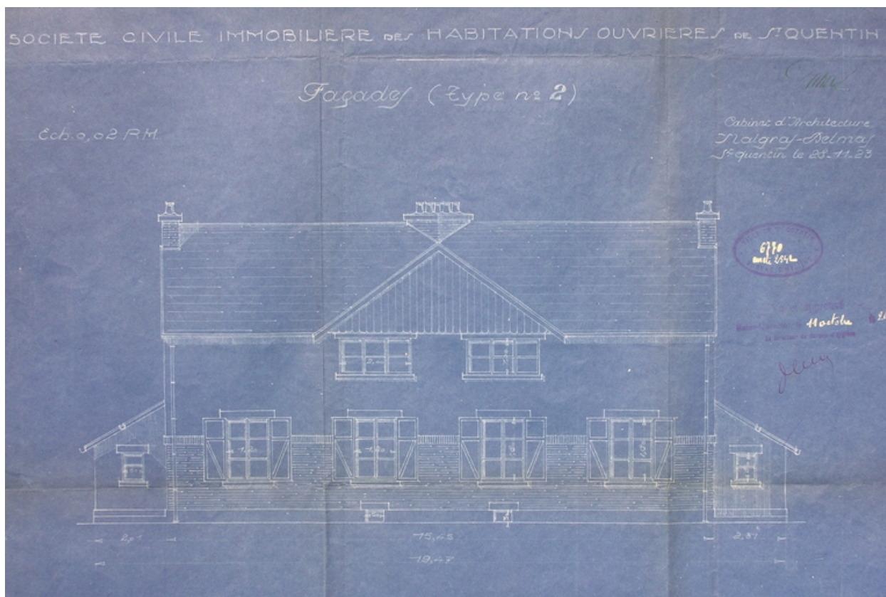
Façade, par Malgras-Delmas, 1923 (AC Saint-Quentin).
