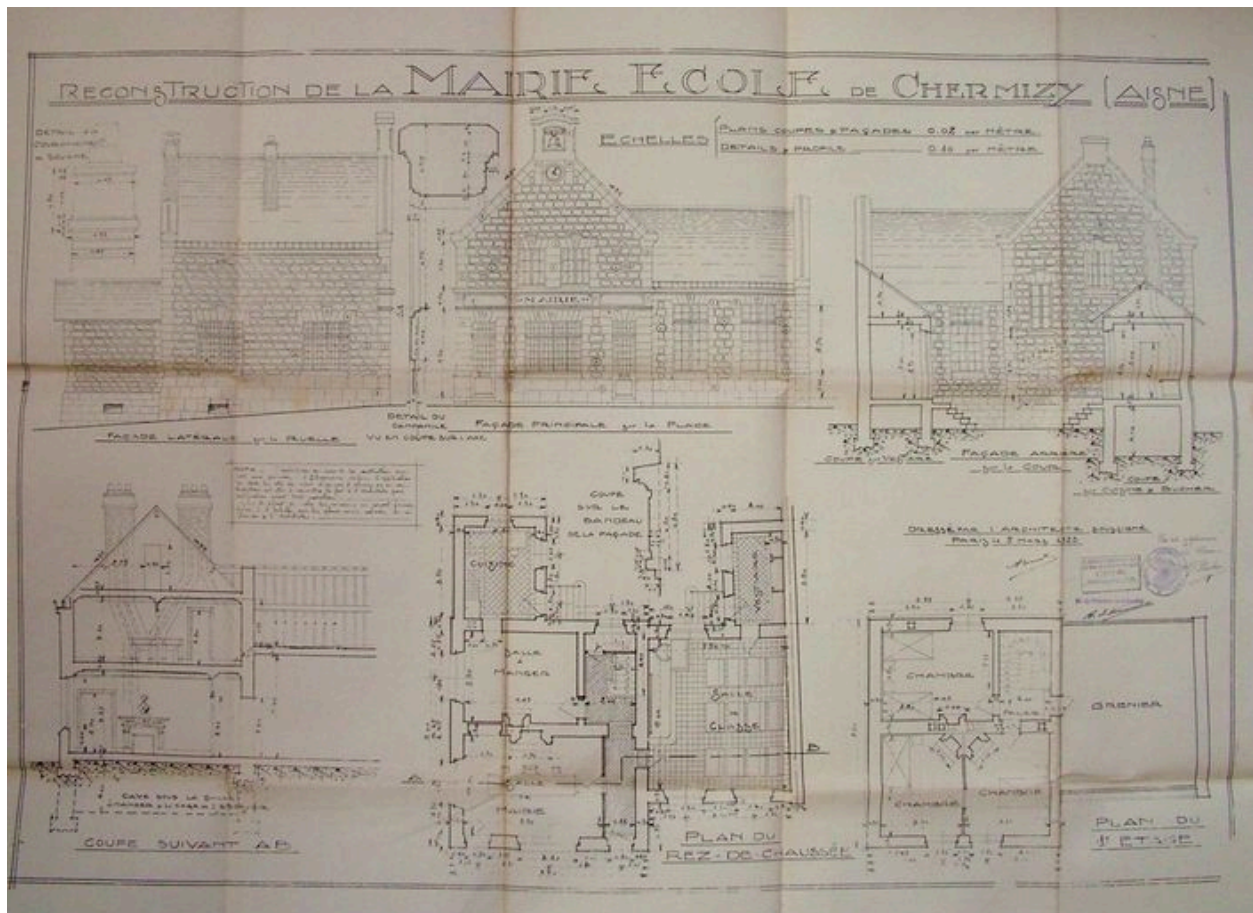
Plan de la mairie-école, par A. Bonnet, en 1923 (AC).
