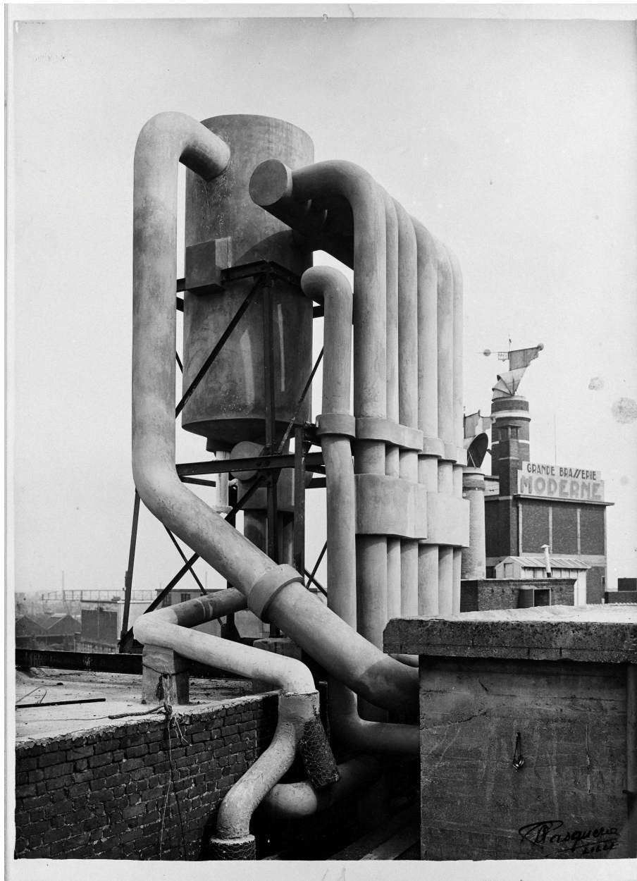
Installation frigorifique extérieure : système flooded (séparateur liquide-gaz) (AP Coutances).
