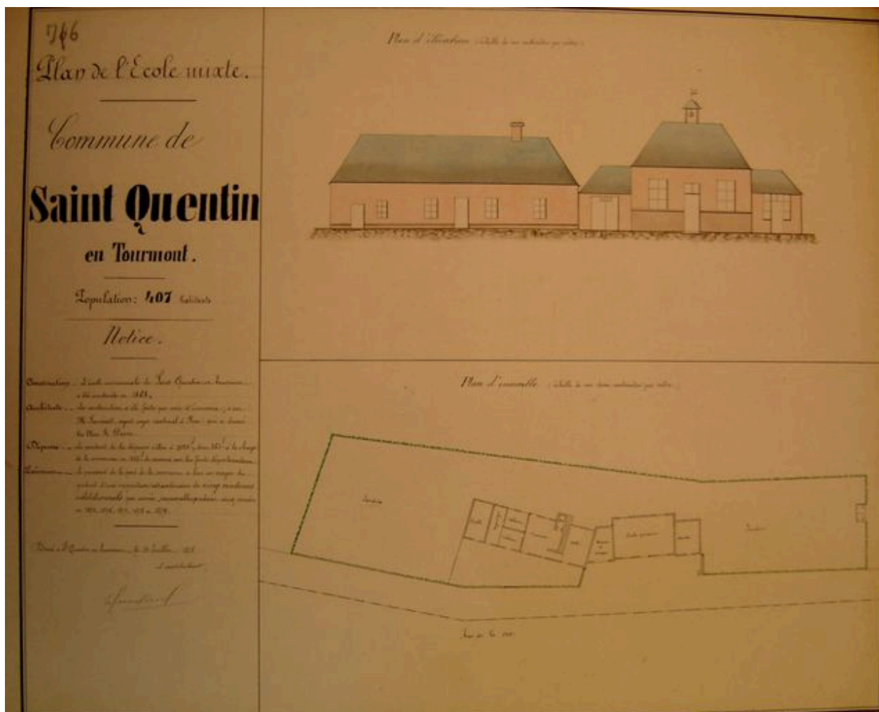
Plan et élévation de l'école mixte en 1878.
