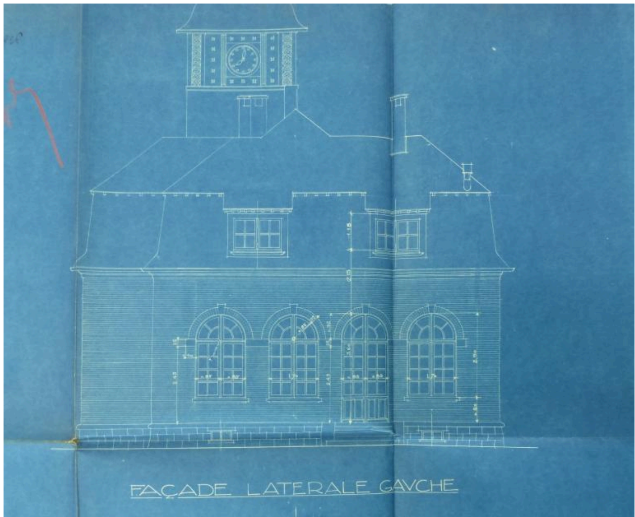
Projet de reconstruction de l'église de Villers-Bretonneux. Somme. Façade latérale gauche. Tirage de plan, A. Guilbert architecte, 22 juillet 1926 (AD Somme ; 99O 3737).
