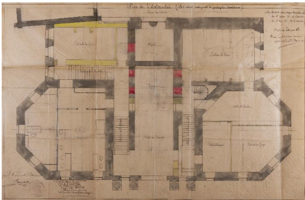
Plan de l'entresol (correspondant au rez-de-chaussée) état avant travaux, Vandembuleke (?) architecte, 1890 (AD Nord, Série 2O 525/87).
