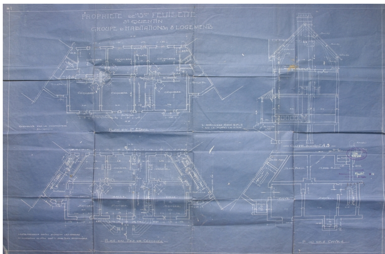
Plans par niveau d'un groupe de 3 logements, par Schneider, 1925 (AC Saint-Quentin).
